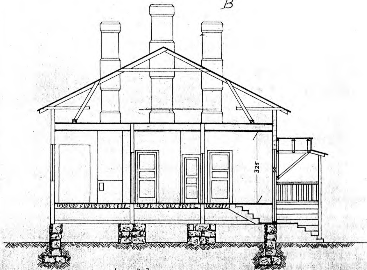
Leikkaus A-B.
