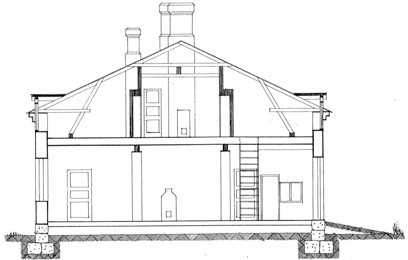
Leikkaus A-A
